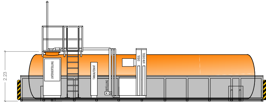
ANSICHT LÄNGS
