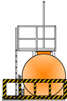
ANSICHT QUER
